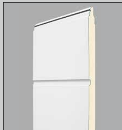
Prierez sekcionálnej garážovej brány
