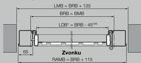
Horizontálny rez
